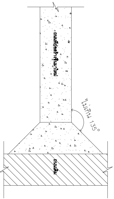
แบบแสดงการเชื่อมต่อระหว่างถนนเดิมกับถนนที่ทำการก่อสร้างขึ้นมาใหม่
