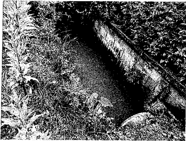
ภาพรางระบายน้ำก่อนดำเนินการขุดลอกดินและต้นไม้
